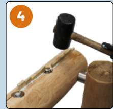
Holzkeile einschlagen
